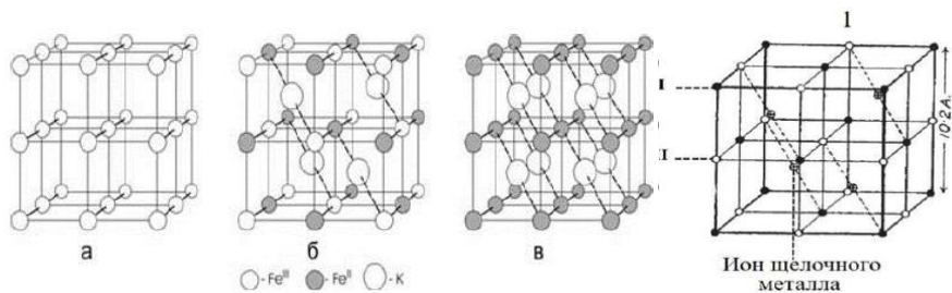
Схемы структуры 2-3 из литературы [4], [5]
