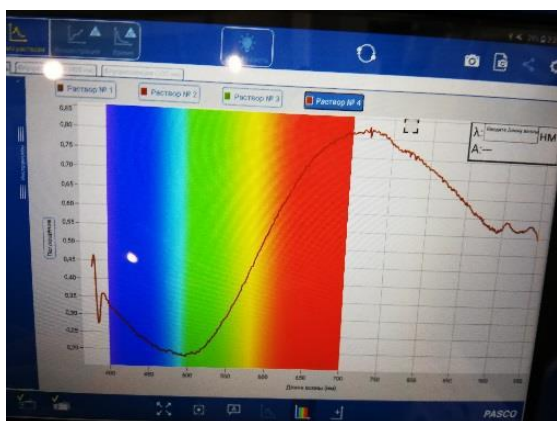
Рис.13. Кривая поглощения раствора
