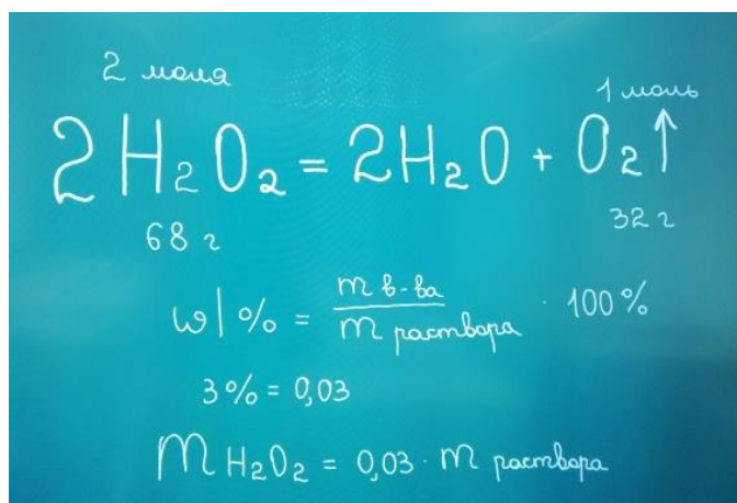
Рис.21. Расчёты по уравнению
