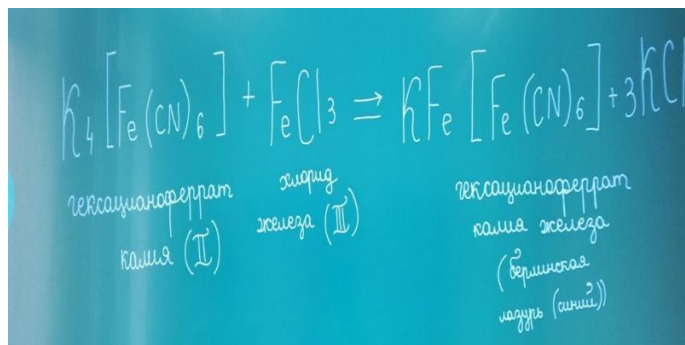
Рис.3. Уравнение реакции
