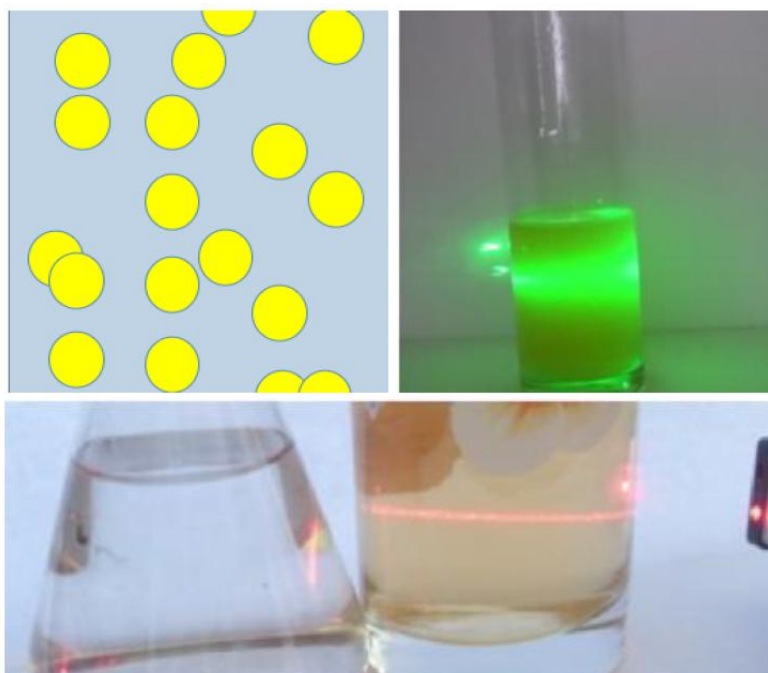
Рис.1. Методика исследования золь
