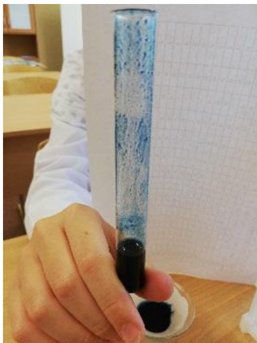
Рис.4. Золь берлинской лазури
