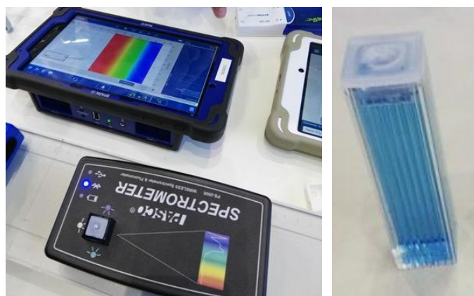
Рис.14. Спектрофотометр
