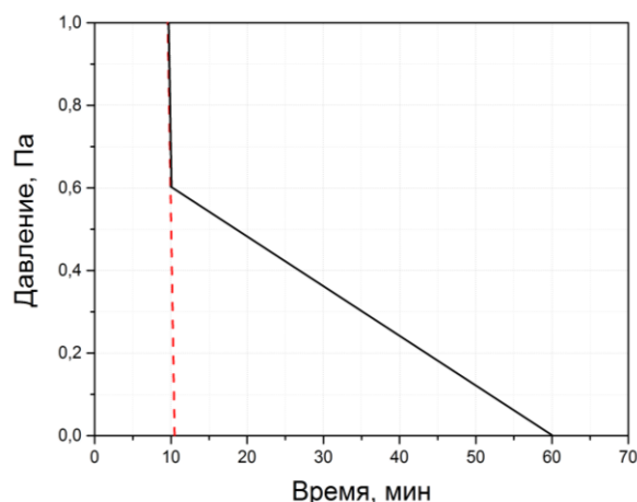
Рис. 2. Зависимость давления в рабочей камере от времени. Пунктирная линия соответствует вакуумированию пустой камеры, а сплошная – этой же камеры, содержащей лепесток ромашки
